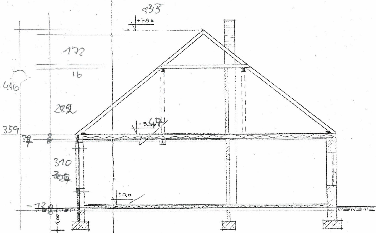
SCHNITT
